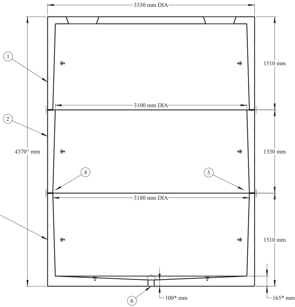
SECTION A-A
